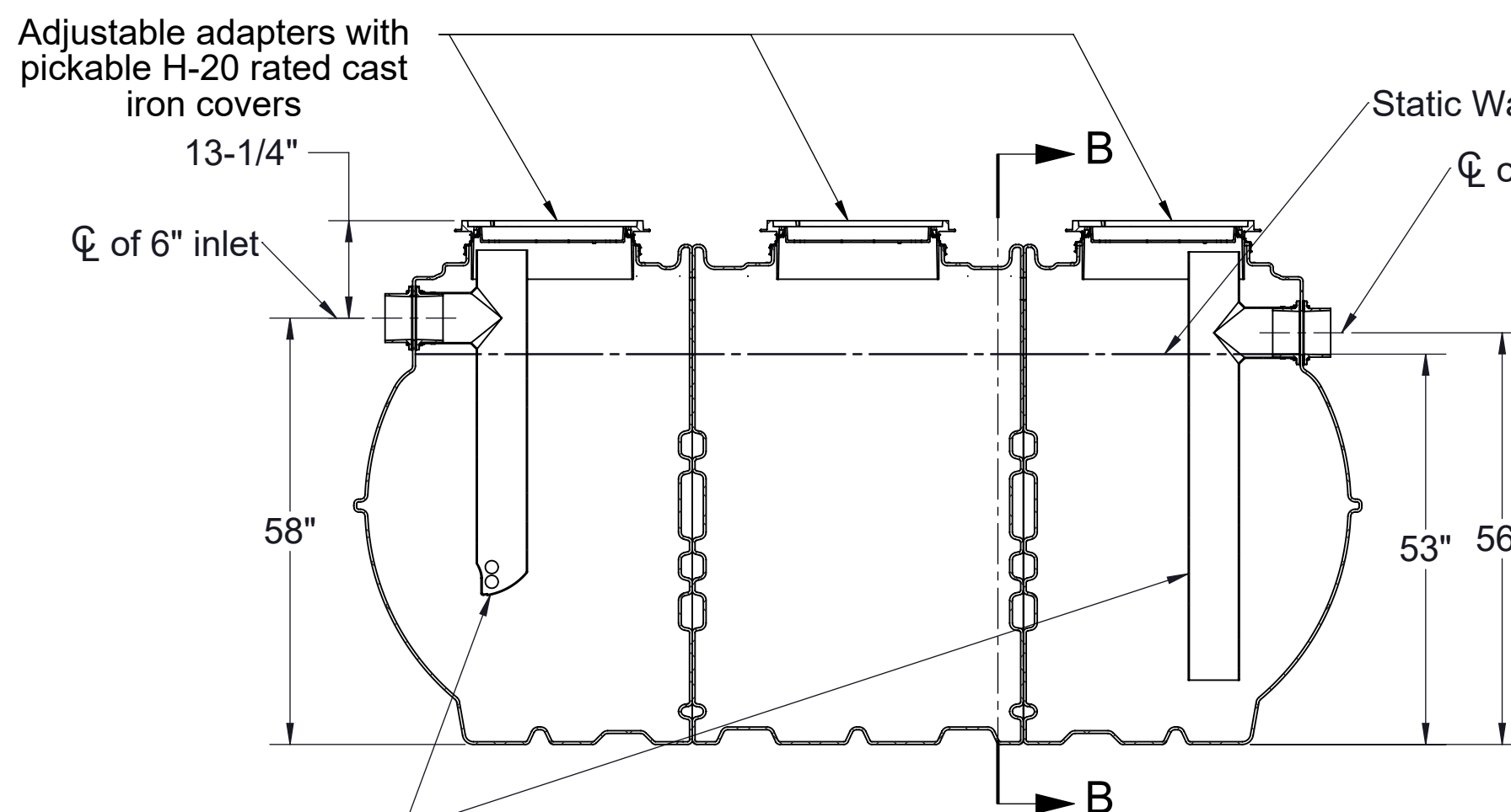
SECTION A-A
