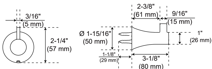
Robe Hook
