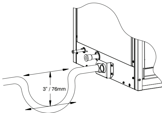
Fig. 15 - Condensate Trap
