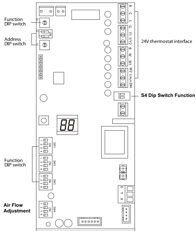
Fig. 14 — 24 Volt Interface
