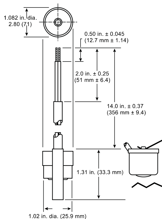
Fig. 10 Aquastat dimensions
