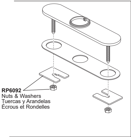
RP71451▲ Optional 10" Escutcheon with 8" Centers, Mounting Screws and gasket (not included) Chapa opcional de 10" de 8" centros, Tornillos para la Instalación y Empaque (no incluido) Plaque de finition facultative de 10 po pour 8 po centres, vis de montage, écrous, rondelles et joint (non inclus)
