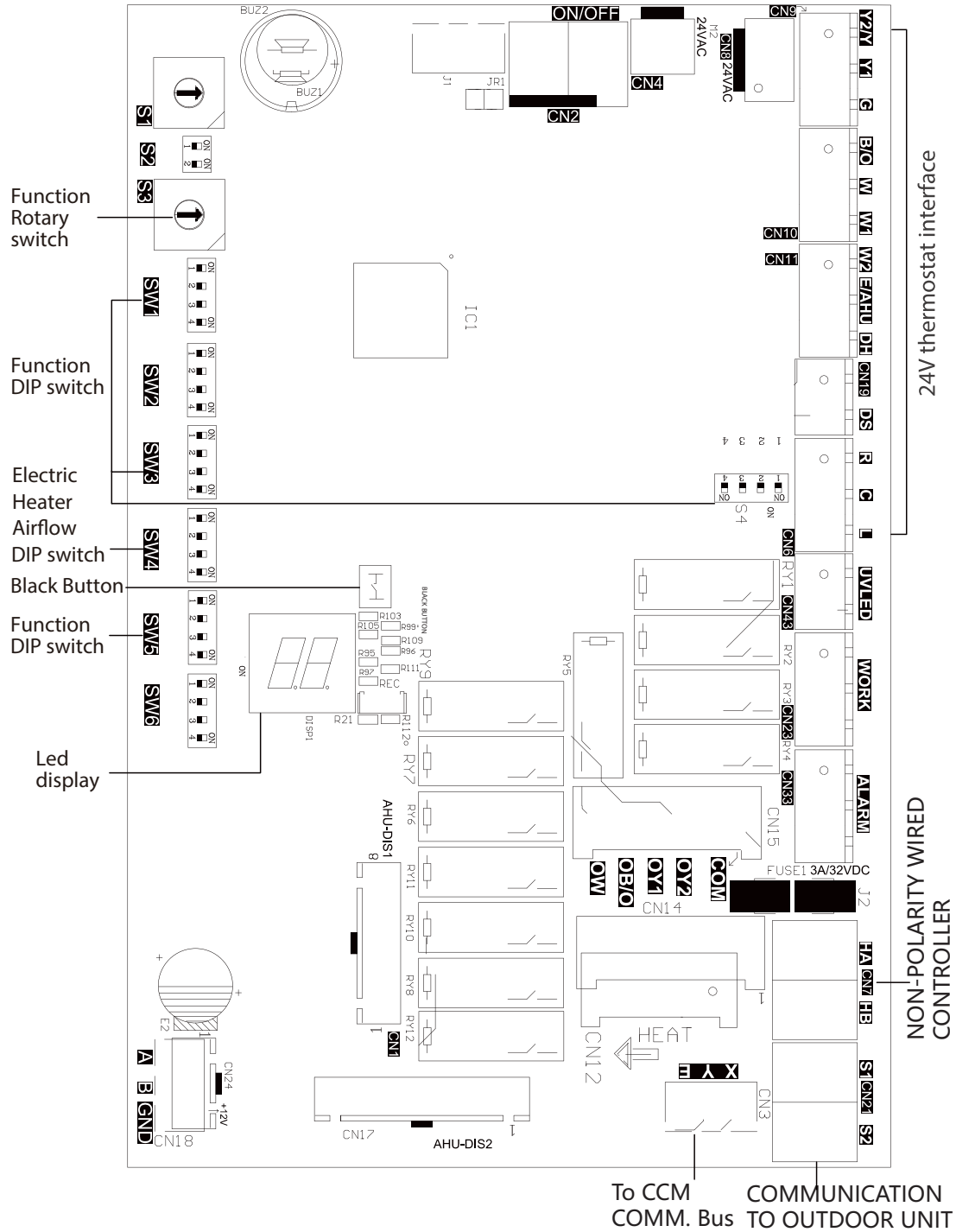
Fig. 10 – 24 Volt Interface
