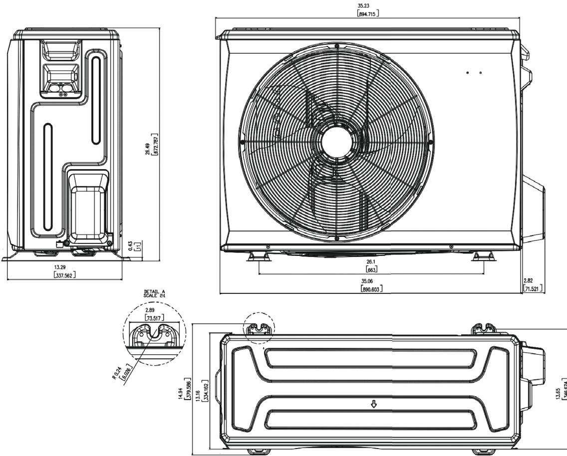
Fig. 3 – Size 18K
