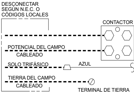
Fig. 8 – Conexiones de tuberías
