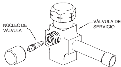
Fig. 5 – Válvula de servicio de vapor
