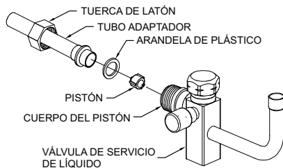
Fig. 4 – Válvula de servicio de líquidos con pistón de calefacción y tubo adaptador
