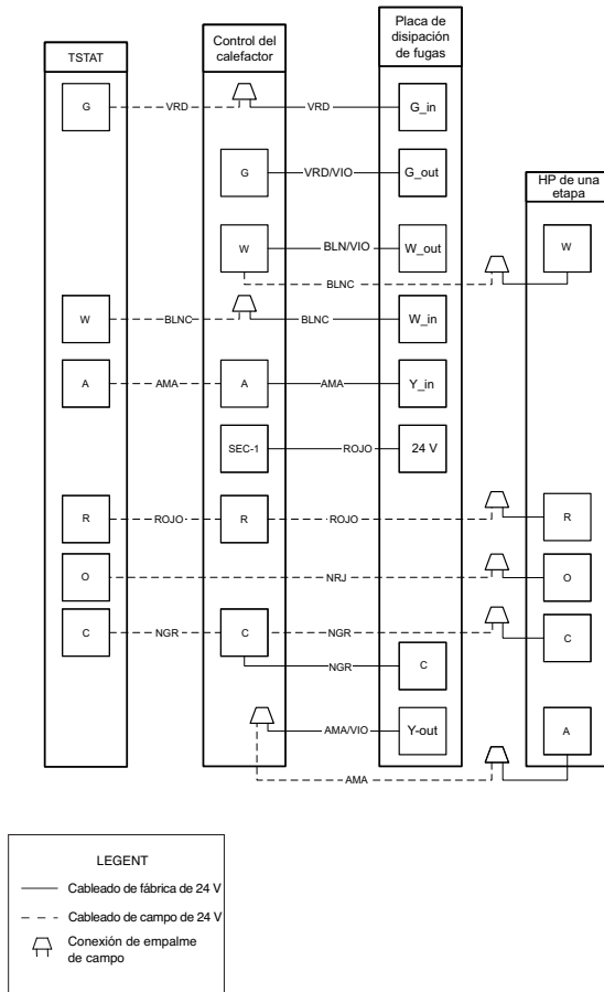
Fig. 10 – Diagrama de cableado genérico (Consulte las instrucciones de instalación del termostato para conocer las combinaciones de unidades específicas)
