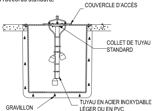
SUPPORT TYPIQUE DE FLOTTEUR POUR COUVERCLE DE PUITS EN ACIER
