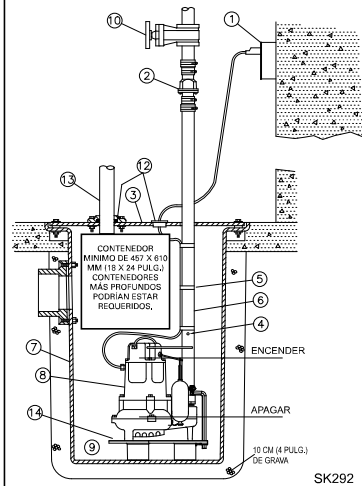
INSTALACIÓN TÍPICA PARA ACHIQUE
