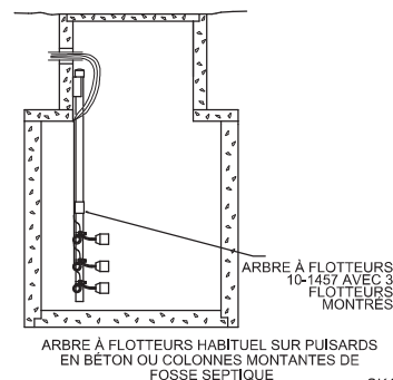
ARBRE À FLOTTEURS HABITUEL SUR PUISARDS EN BÉTON OU COLONNES MONTANTES DE FOSSE SEPTIQUE
