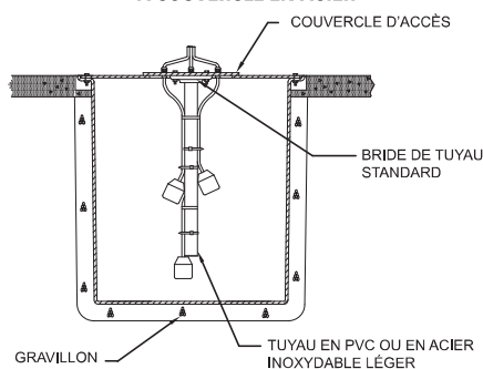
ARBRE À FLOTTEURS HABITUEL SUR PUISARDS À COUVERCLE EN ACIER
