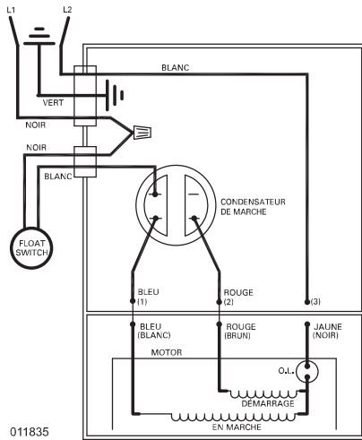
SCHEMA DE CÂBLAGE POUR MODÈLES
