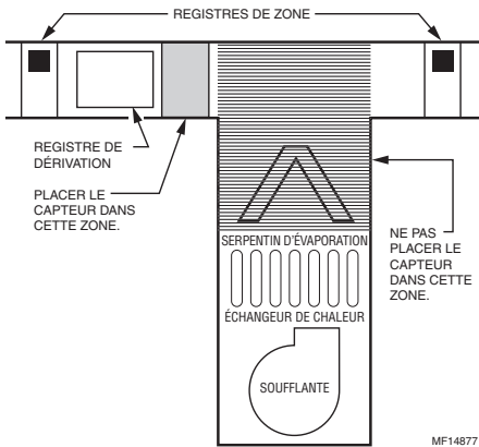
Fig. 2. Emplacement de montage du capteur de température d'air de gaine.
