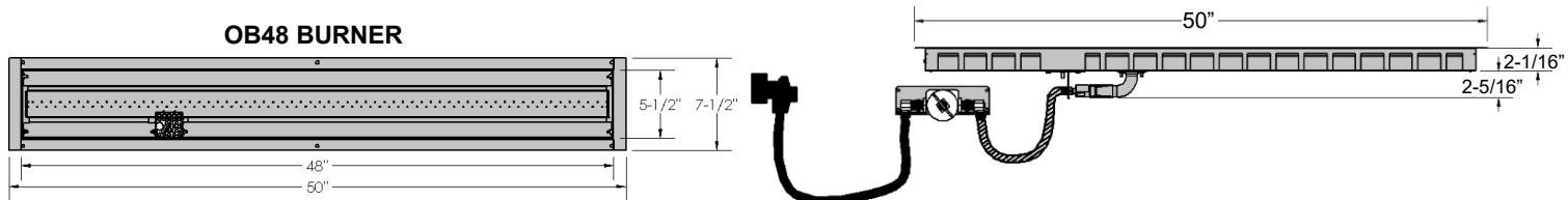
OB72 BURNER
