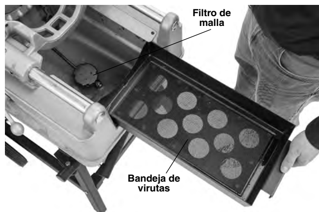
Figura 30 – Extracción de la bandeja de virutas
