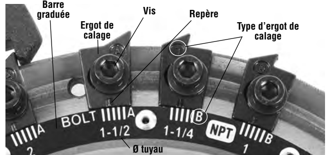
Figure 15 – Réglage du filetage
