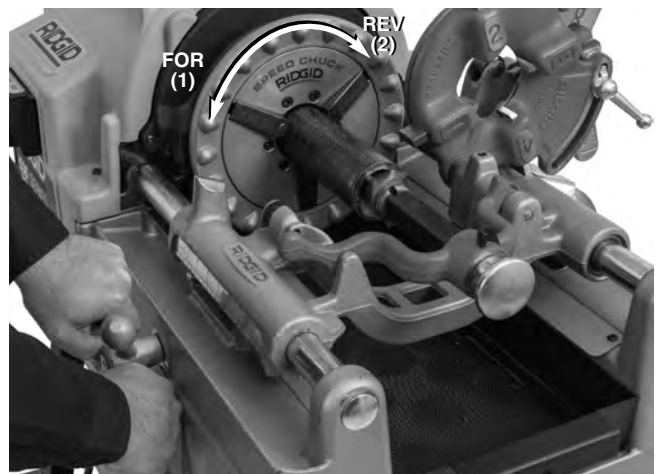
Figure 22 – Alésage du tuyau avec la machine en marche
