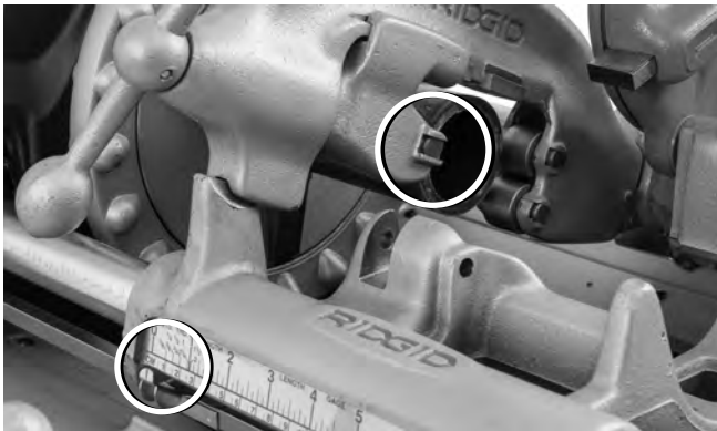
Figure 20A – Lame du galet de coupe appuyée contre l'extrémité du tuyau. Curseur à « 0 ».
