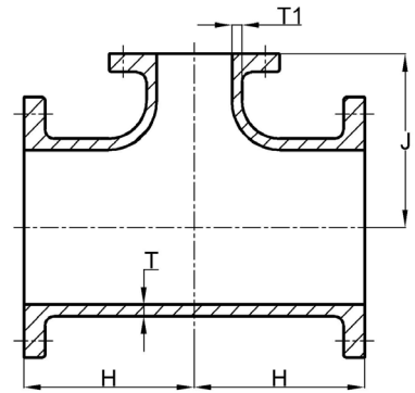
DFT
