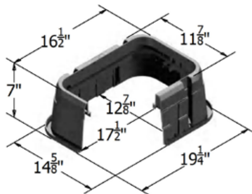
1015-06 HDPE
