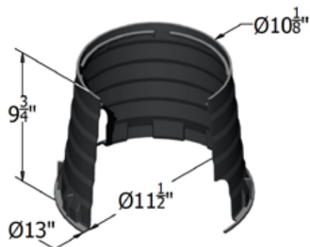
0011-10 HDPE
