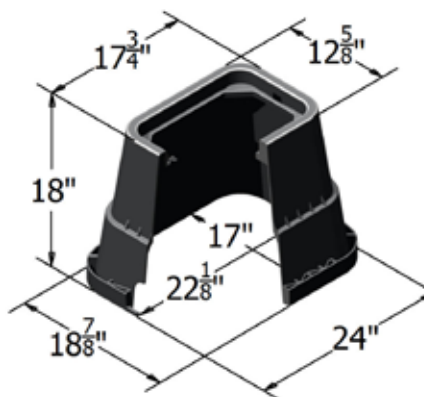
1520-18 HDPE
