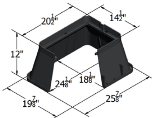
0012-12 BODY HDPE
