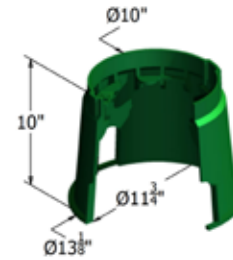
0910-10 HDPE
