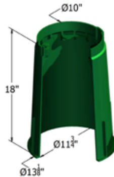
0910-18 HDPE
