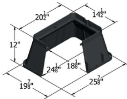
0012-12 BODY HDPE
