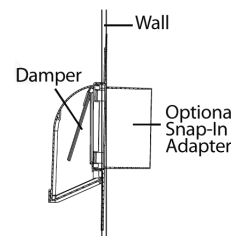
WC28 - Wall Cap vent
