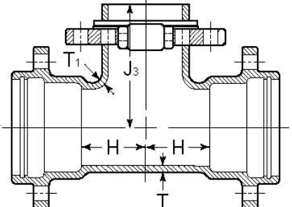
UTxSwivel Tee
