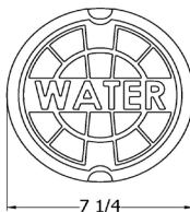
1 1/8" Lid
