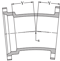
11 1/4° (1/32) MJxFE
