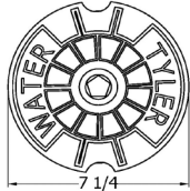
Lock Lid
