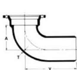
90° Bend
