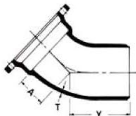
45° Bend
