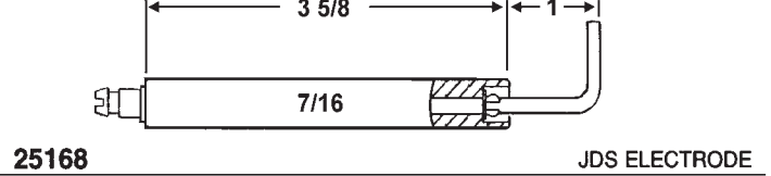
25158 TYPE 33 PILOT SPARK ROD Midco 6430-00
