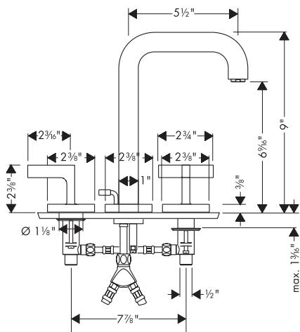
39133XX1 / 39135XX1
