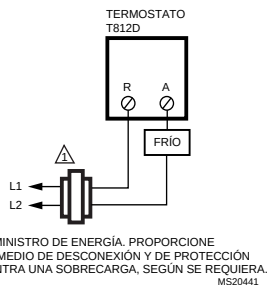
Fig. 8. T812D en aplicación de enfriamiento únicamente.
