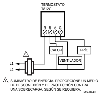
Fig. 7. T812C en sistema de calefacción y enfriamiento.
