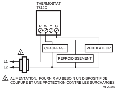
Fig. 7. T812C dans un système de chauffage et de refroidissement.
