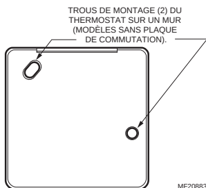
Fig. 2. Emplacement des trous de montage sur les modèles sans plaque de commutation.
