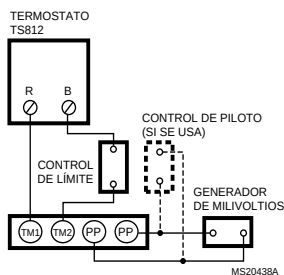
Fig. 5. Conexión típica al TS812A en sistema de milivoltios.
