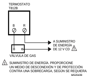
Fig. 6. T812B en aplicación de 12 V cd.
