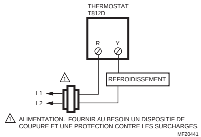
Fig. 8. T812D dans une application de refroidissement seulement.
