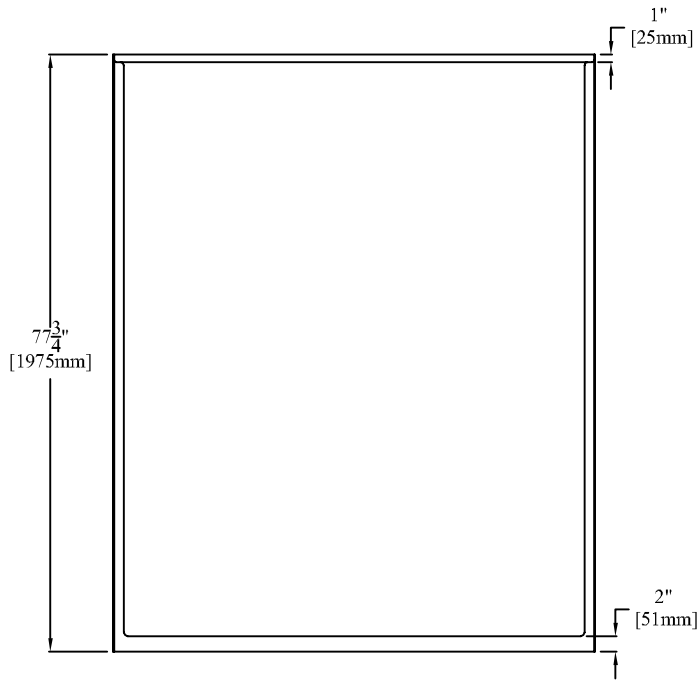
ELEVATION
