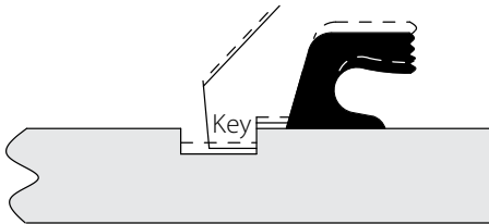
Eccentric Groove
