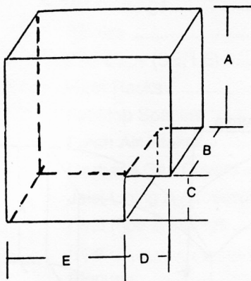
FIG. 3 ELBOW 90° SQUARE HEEL & THROAT
