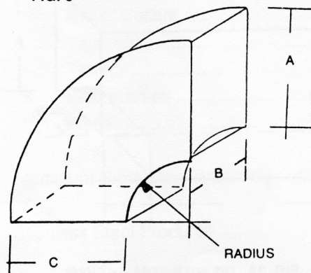
FIG. 7 90° ELBOW RADIUS HEEL & THROAT
