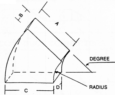
FIG. 10 ELBOW RADIUS HEEL & THROAT
