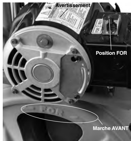
Figure 8 – Rotation du tambour en position FOR (marche avant)
