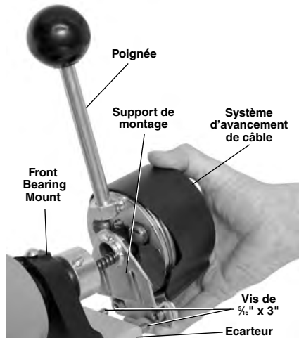
Figure 5 – Montage du système d'avancement de câble sur le cadre
