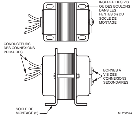
Fig. 10. Montage sur socle du transformateur AT87.
