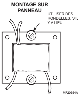
Fig. 1. Insérer des boulons dans les fentes pour un montage sur panneau.
