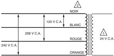
Fig. 11. Schéma du transformateur AT20/AT40
