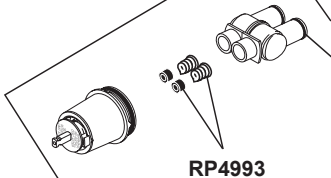
RP4993 Seats & Springs Asientos y Resortes Sièges et Ressorts
