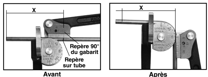
Figure 4A – Alignement pour ceintrage à 90° à gauche
