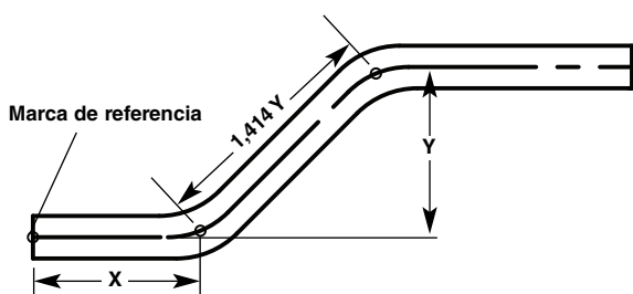
B – Tubo doblado con marcas
