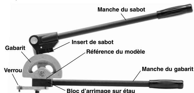
Figure 1 – Ceintreuse de plomberie série 300
