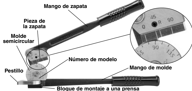
Figura 2 – Dobladora de la serie 400 para plomería
