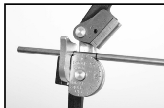
Figura 3 – Colocación del tubo en la dobladora
