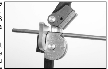
Figure 3 – Positionnement du tube dans a ceintreuse
