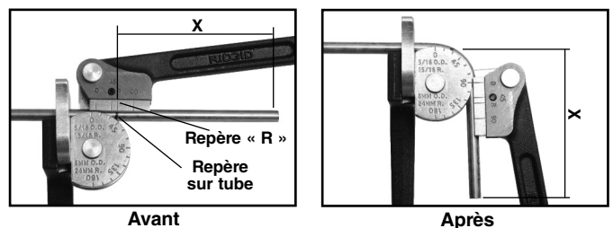
Figure 4B – Alignement pour ceintrage à 90° à droite
