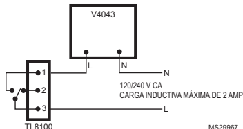
Fig. 5. Diagrama de cableado de una válvula de voltaje de línea (V4043 o similar).
