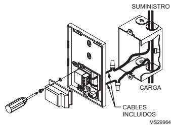
Fig. 2. Trazado de los cables hacia el termostato.
