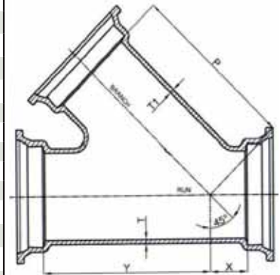
Wyes Lateral 45°
