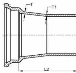
MJ x PE (large end MJ)
