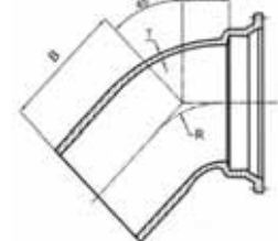
MJ x PE Bend 45°
