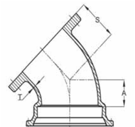
MJ x Flange 45° Bend
