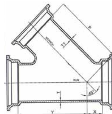
Wyes Lateral 45°
