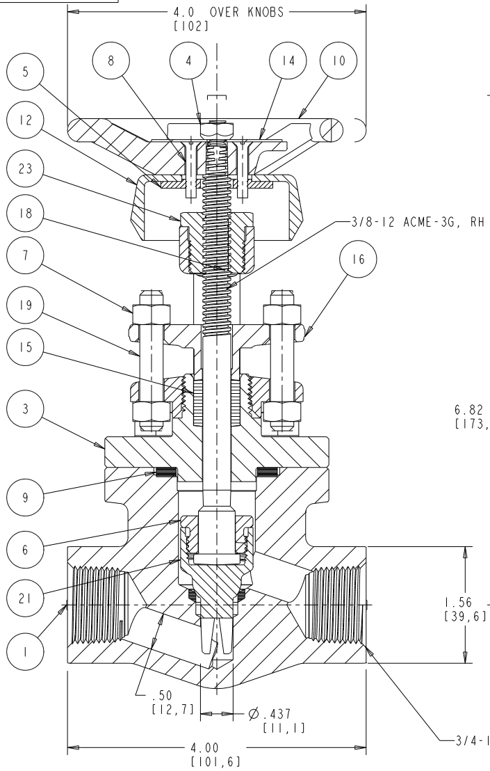
SECTION A-A
