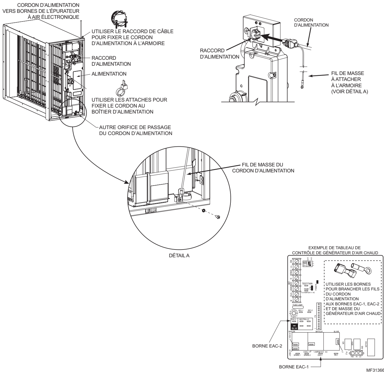
Fig. 15. Connexions électriques.
