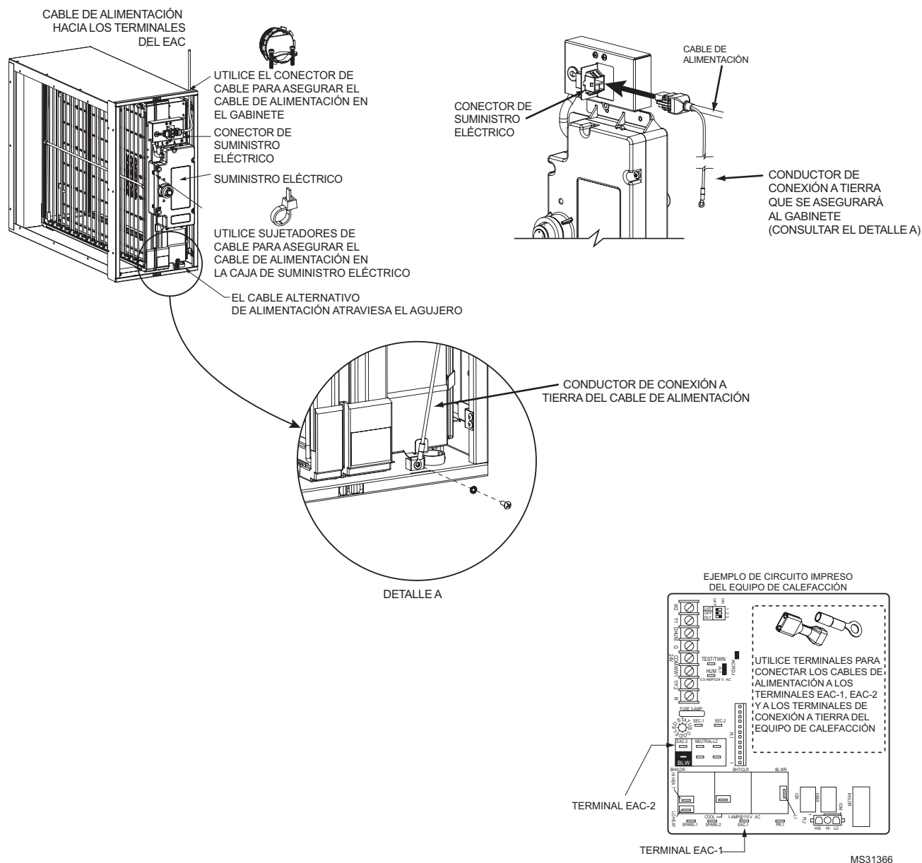
Fig. 15. Conexiones eléctricas.
