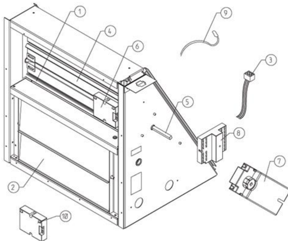
RXRD-MECM3 Assembly
