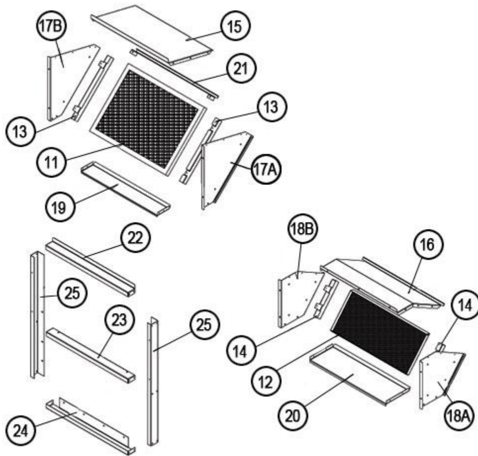
RXRD-MECM3 Hood
