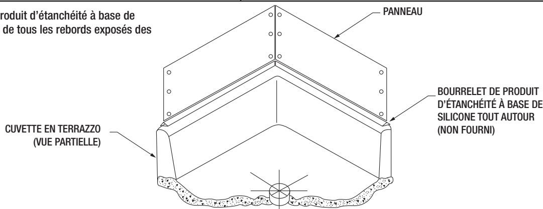
SUPPORT ANGULAIRE
