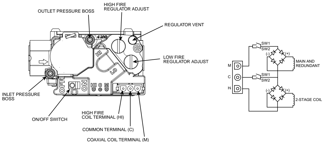
Fig. 4 – Mate-N-Lok wiring
