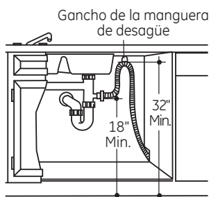
Instalación de la T de desechos
