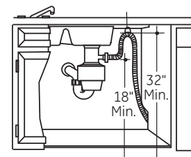
Instalación del eliminador de desechos
