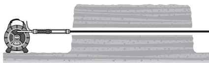
Figura 11 – Conecte la manguera de aire al Sistema de inspección CROSSCHEK
