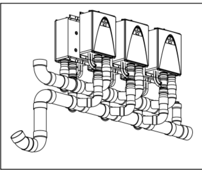
Figure 13. Configuration horizontale (dos à dos)
