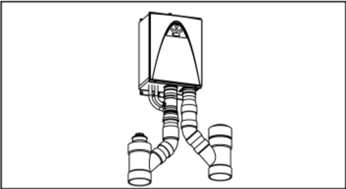
Figure 23. Configuration verticale (gainés ou puits séparés)
