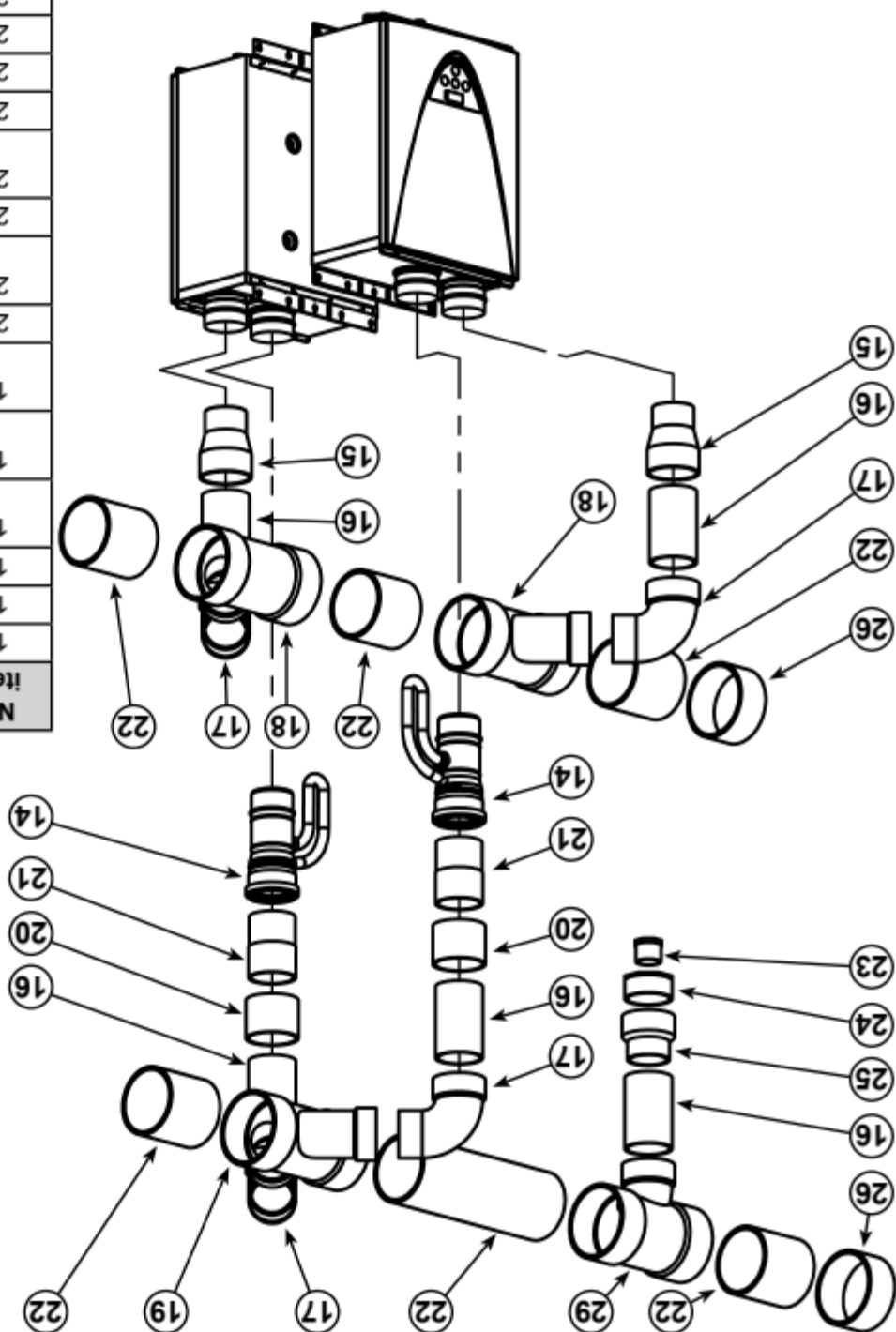
Figure 12. Composantes, configuration horizontale (dos à dos)
