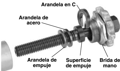
Figura 2 – Ensamblaje de la Cortadora: oriente las arandelas en C y de acero con su parte biselada hacia la Superficie de empuje
