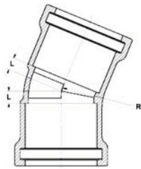
22 1/2 Bend
