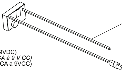
060968A Battery Box Extension Cable Câble de rallonge du boîtier des piles Cable de extensión del receptáculo de las pilas
