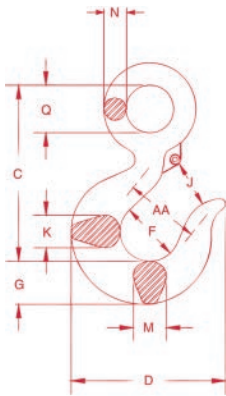
L-320 EYE HOOK
