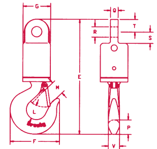
S-6 Eye & Hook
