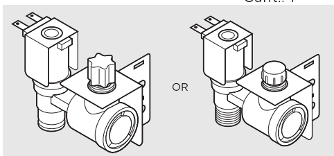
Válvula de agua Cant.: 1
