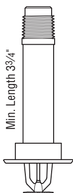
63-101-X-XXX w/Std. Escutcheon
