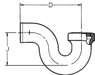
TAP P-TRAP
