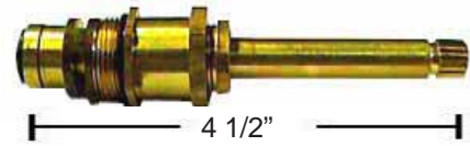
SA412 Diverter Ea.
