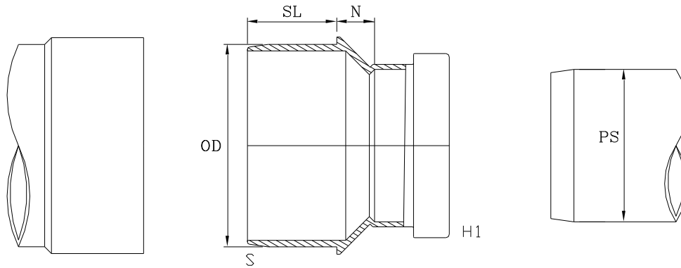
GASKET OR SW SEWER HUB GASKET OU SW EGOUT FEMELLE
