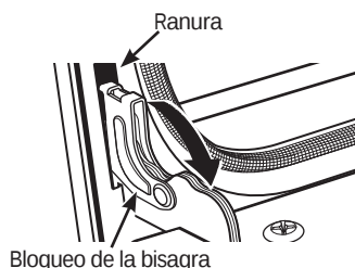
Bloqueo de la bisagra Empuje los bloqueos de la bisagra hacia abajo para desbloquear
