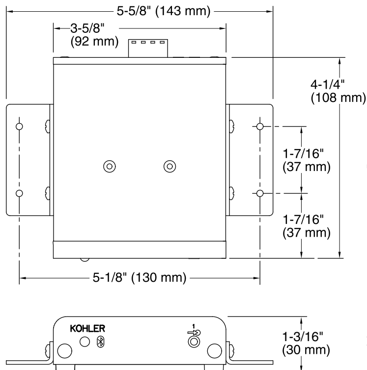
Amplifier Module
